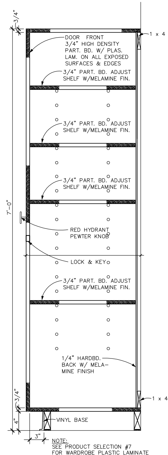
3 A1.5 WARDROBE CAB. SCALE: 1" = 1'-0"
