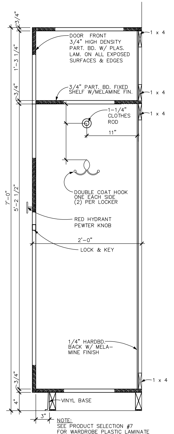
4 A1.5 WARDROBE CAB. SCALE: 1" = 1'-0"
