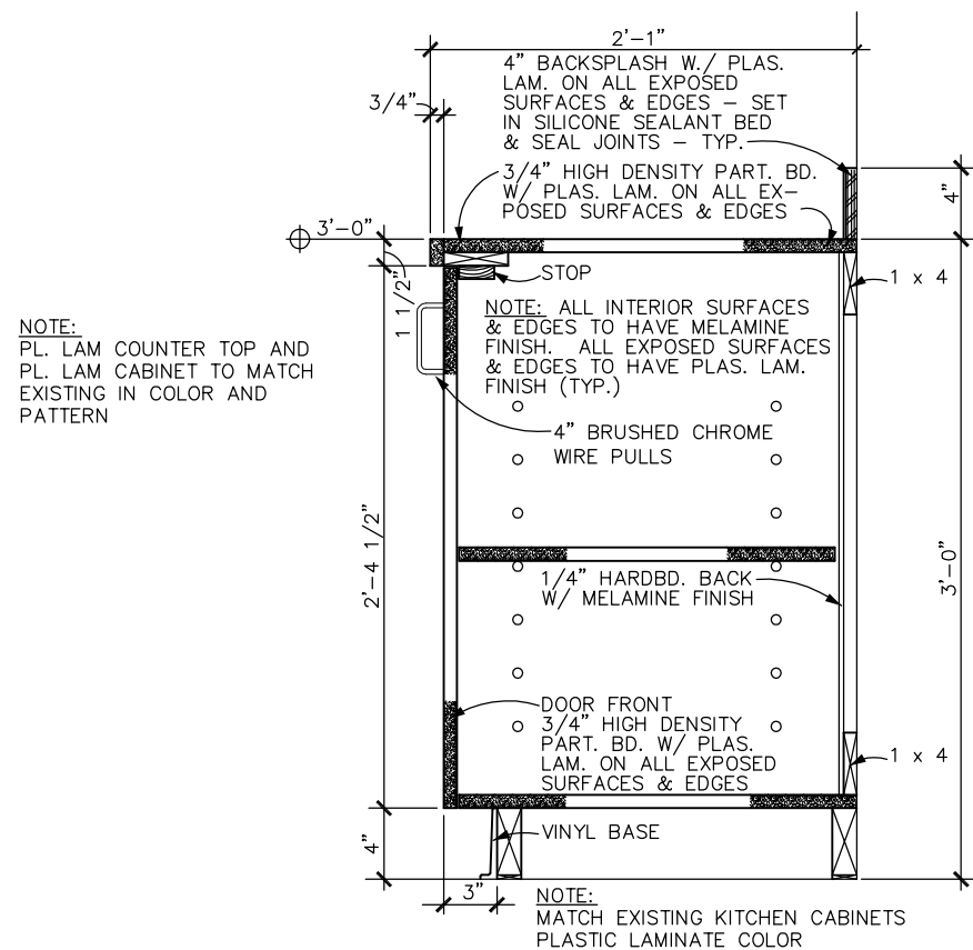
2 A1.5 BASE CABINET SCALE: 1" = 1'-0"
