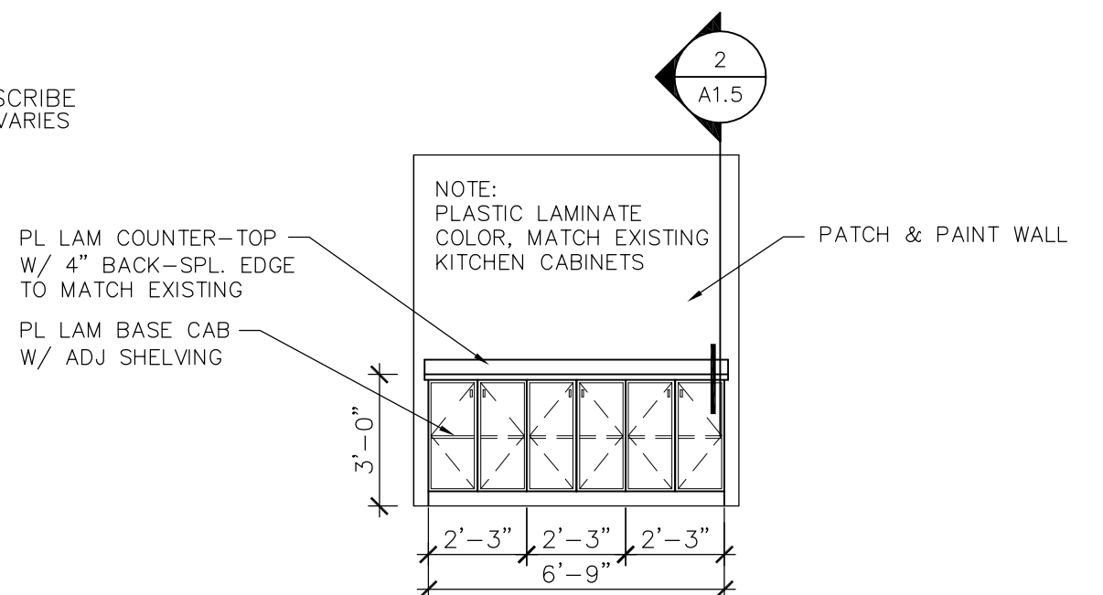
3 A1.4 DINING 135 SCALE: 1/4" = 1'-0"
