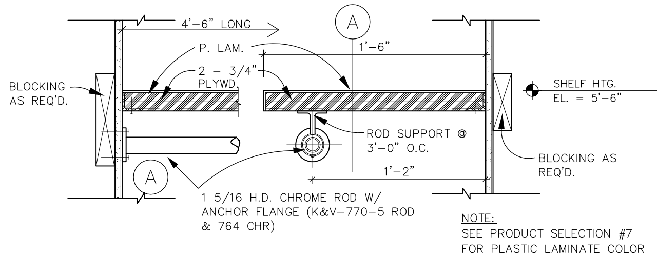
1 A1.5 COAT SHELF & ROD SCALE: 1-1/2" = 1'-0"
