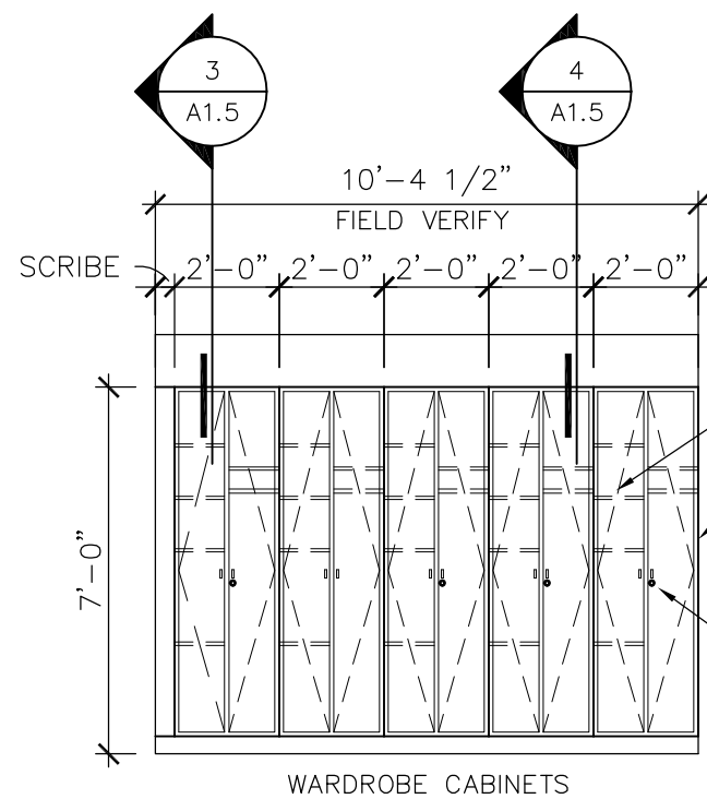
1 A1.4 SHOWER RM 126 SCALE: 1/4" = 1'-0"
