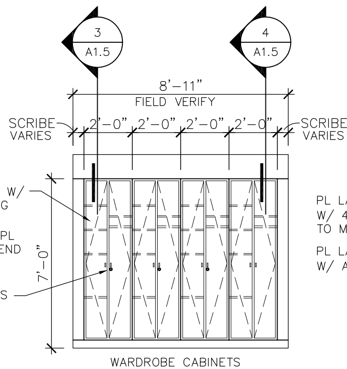
2 A1.4 BEDRM 131A,B,C&D SCALE: 1/4" = 1'-0"
